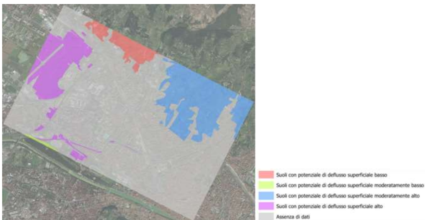
Figura 6-7 Gruppo idrologico USDA (Fonte: Regione Toscana)
