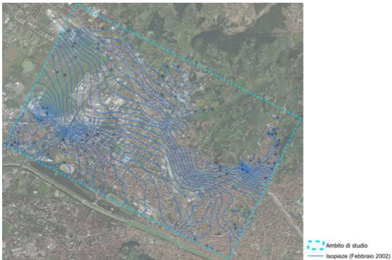
Figura 6-15 Carta delle isopieze – quadrante sud-est (Fonte: Comune di Firenze)
