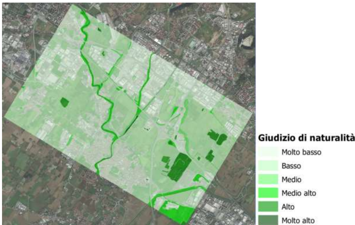
Figura 5-3 Grado di Naturalità del territorio – quadrante nord-ovest
