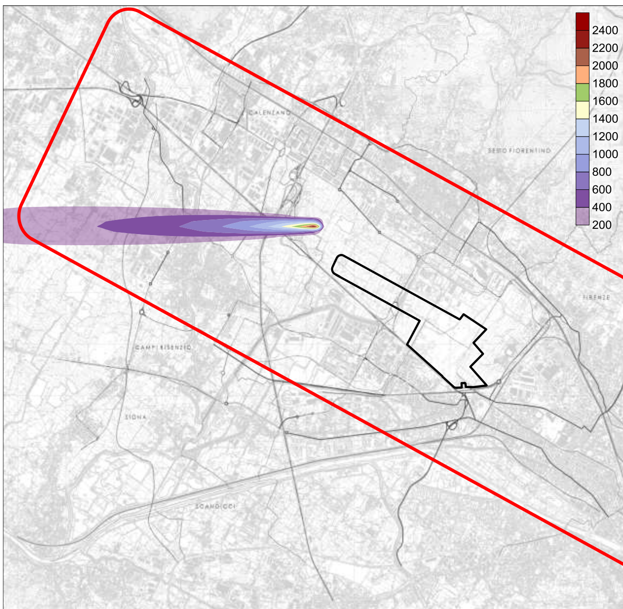
Figura 8 Valori di concentrazione, espressi in \mu\text{g}/\text{m}^3 , massimi orari calcolati sull'arco di 24 ore per emissioni di CO = Monossido di Carbonio da combustione derivata dall'incendio per il crash dell'aeromobile - scenario 3 - condizioni meteo 5D.
