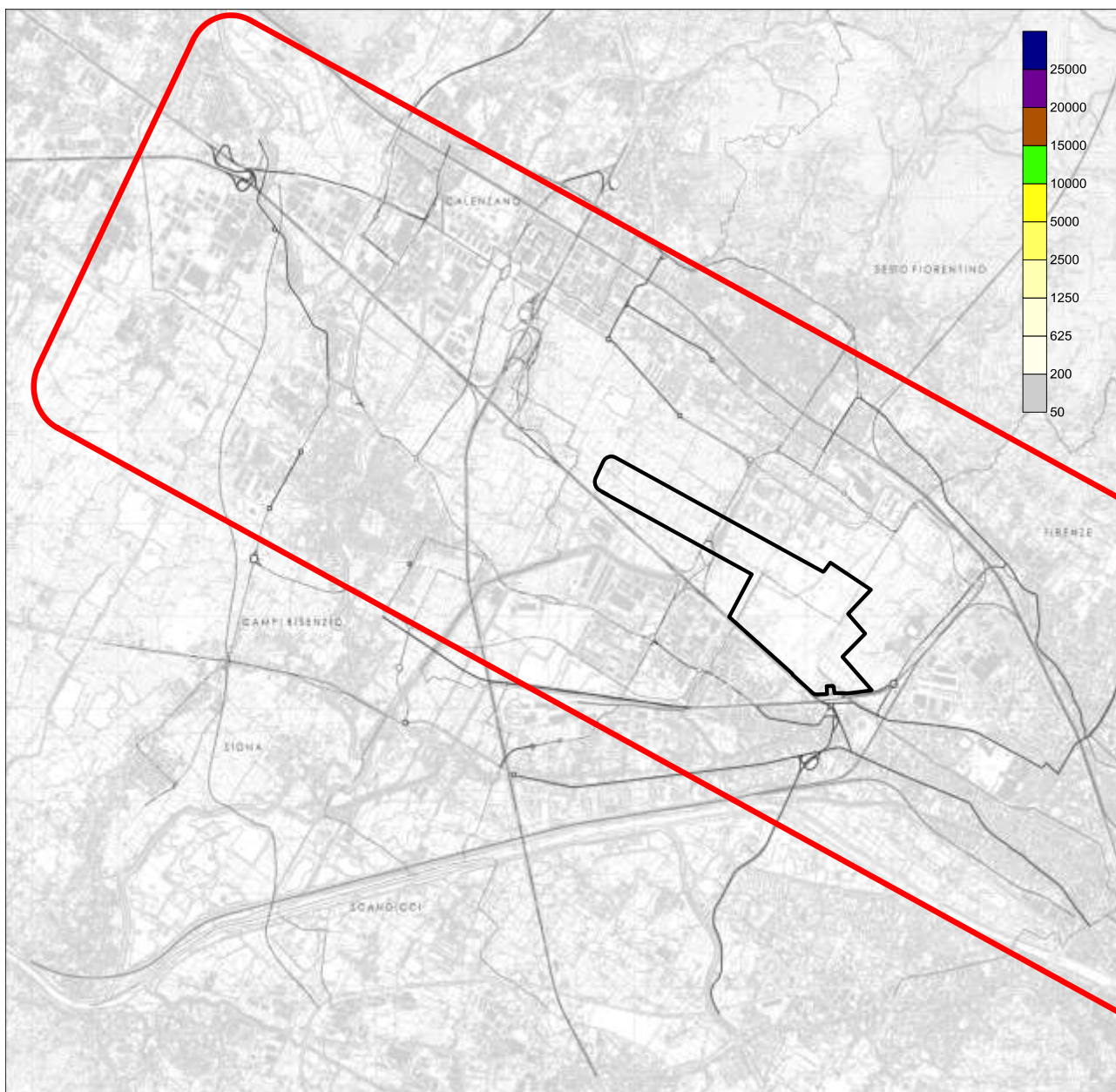
Figura 14 Valori di concentrazione per il quarto intervallo di tempo T4 - 20 minuti a valle dell'evento incidentale, espressi in \mu\text{g}/\text{m}^3 , massimo su media di 20 minuti per le emissioni di soot = particolato Monossido di Carbonio da combustione derivata dall'incendio per il crash dell'aeromobile - scenario 3 - condizioni meteo 2F.
