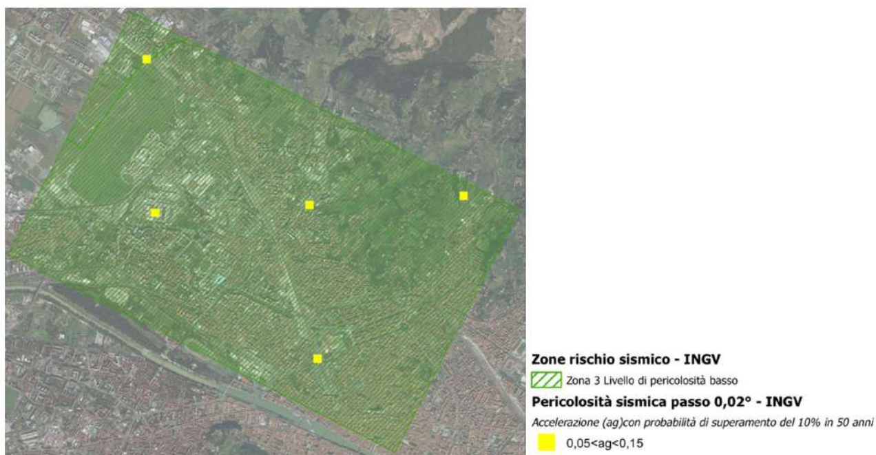
Figura 48 Pericolosità e rischio sismico, quadrante sud est
