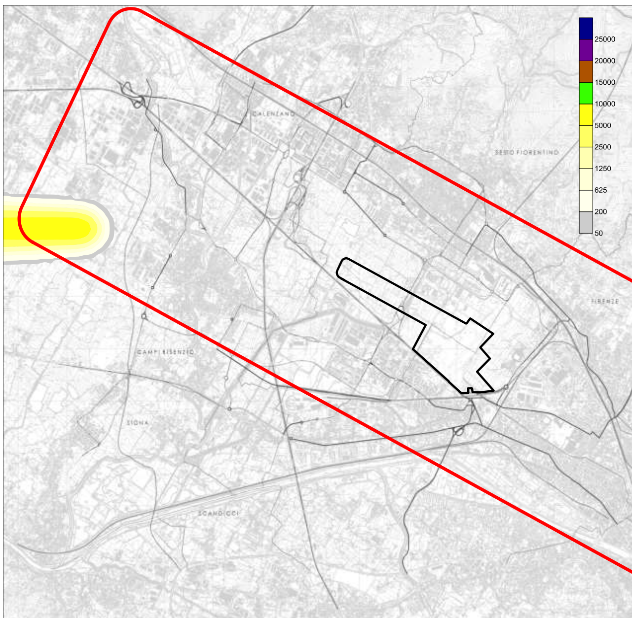
Figura 13 Valori di concentrazione per il terzo intervallo di tempo T3 20 minuti a valle dell'evento incidentale, espressi in \mu\text{g}/\text{m}^3 , massimo su media di 20 minuti per le emissioni di soot = particolato Monossido di Carbonio da combustione derivata dall'incendio per il crash dell'aeromobile - scenario 3 - condizioni meteo 2F.
