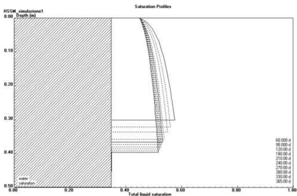
Figura 416 - Scenario II saturazione in acqua della zona vadosa pari al 35 %. Profilo di saturazione relativo ai primi 365 giorni dal rilascio
