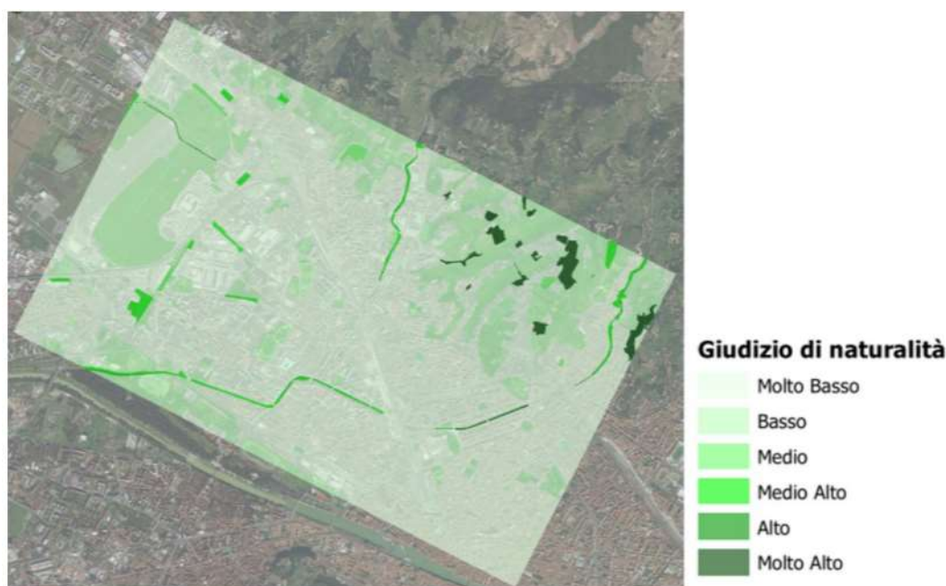
Figura 55 Grado di Naturalità del territorio; Quadrante sud-est
