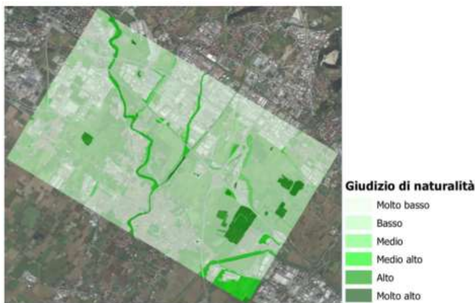
Figura 50 Grado di Naturalità dell'area di studio; Quadrante nord-ovest.
