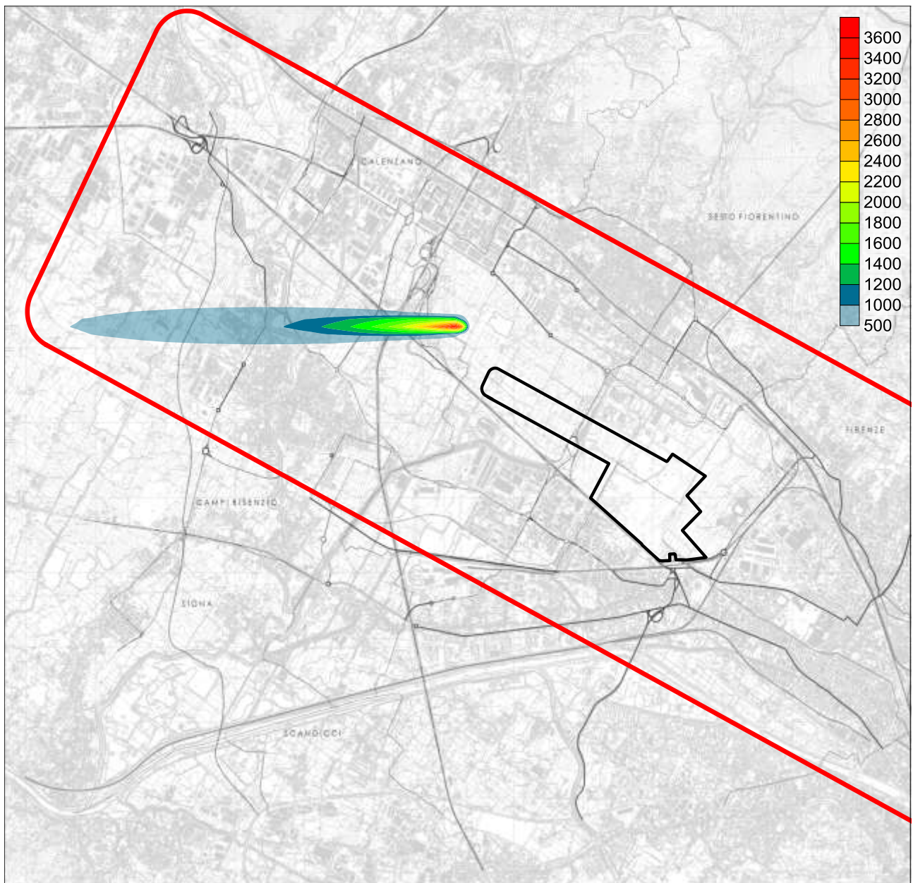
Figura 7 Valori di concentrazione, espressi in \mu\text{g}/\text{m}^3 , massimi orari calcolati sull'arco di 24 ore per emissioni di SOOT = Polveri Totali emesse da fumi della combustione derivata dall'incendio per il crash dell'aeromobile - scenario 3 - condizioni meteo 5D.
